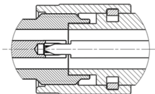
Рисунок 11 – Соединители тип 2,4 мм, 3,5 мм и IX(розетка слева, вилка справа)
